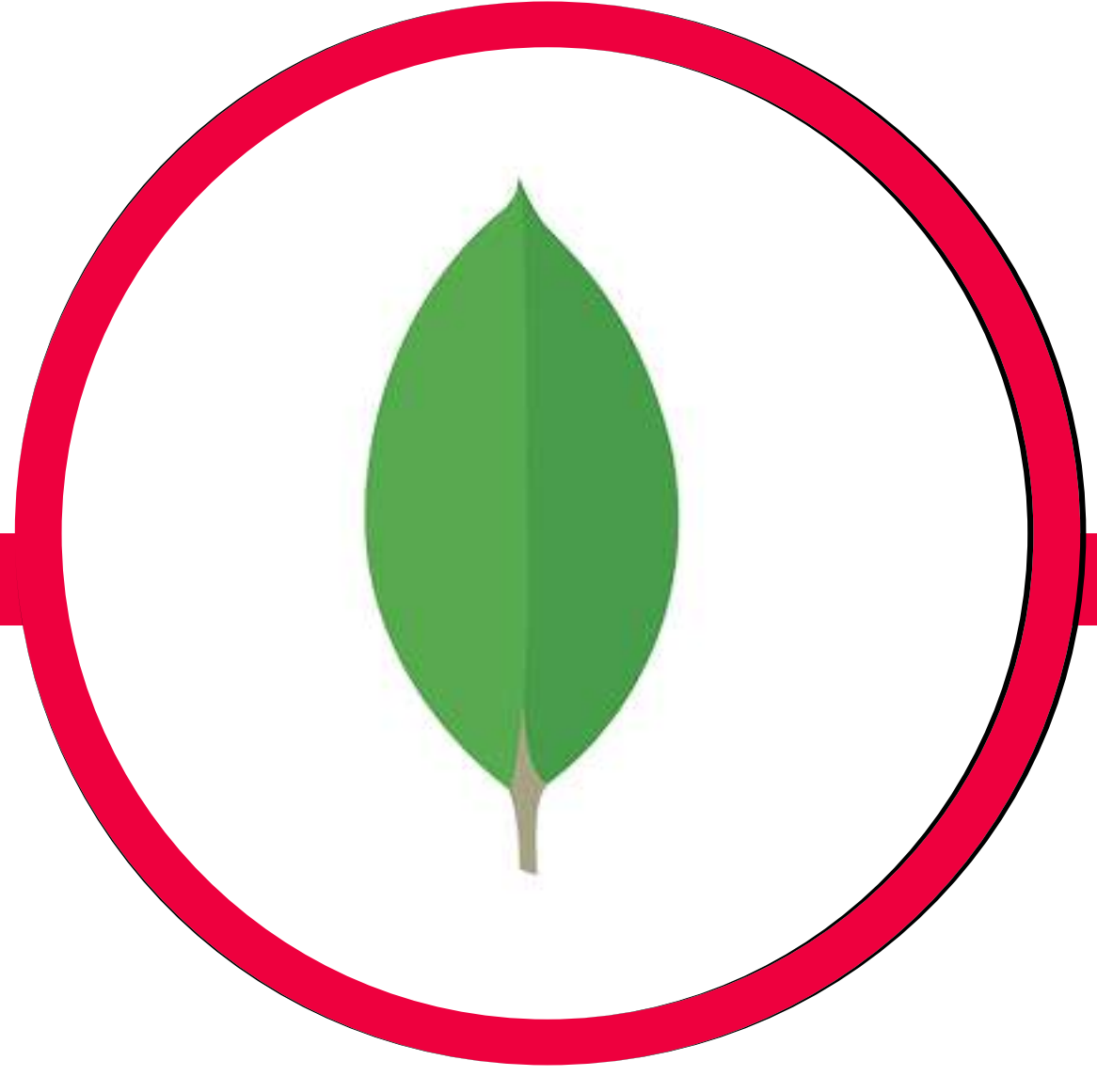
MONGODB
