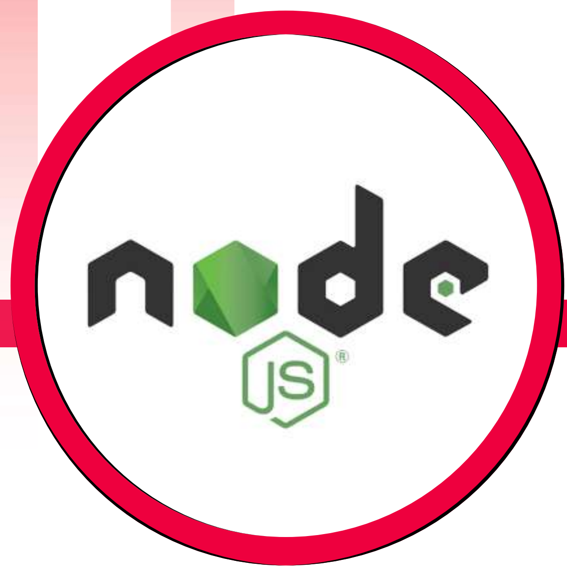
NODEJS
